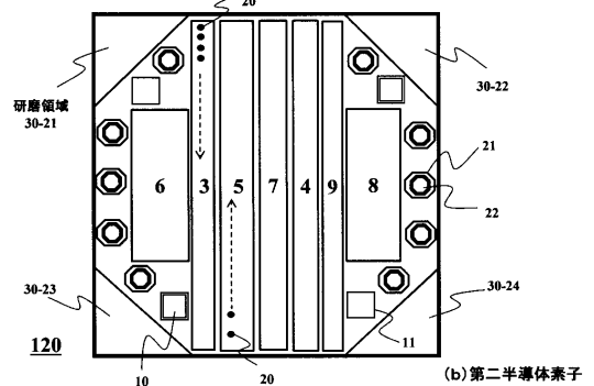
(b) 第二半導体素子
