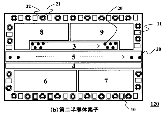
(b) 第二半導体素子
