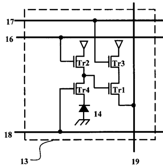
(a) 4トランジスタ画素回路
